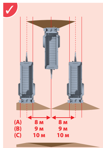
Ширина перекрытия разбрасывания (варируется в зависимости от разбрасываемого материала): (A) 8 м (стандарт) (B) 9 м с ножами (C) 10 м с разбрасывающими дисками
